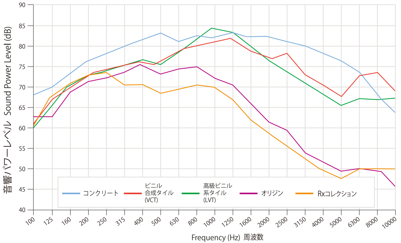
床衝撃音レベル (ASTM E3133に従う)
