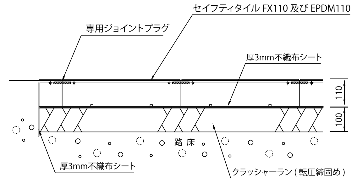
参考施工図 S = 1 / 10
