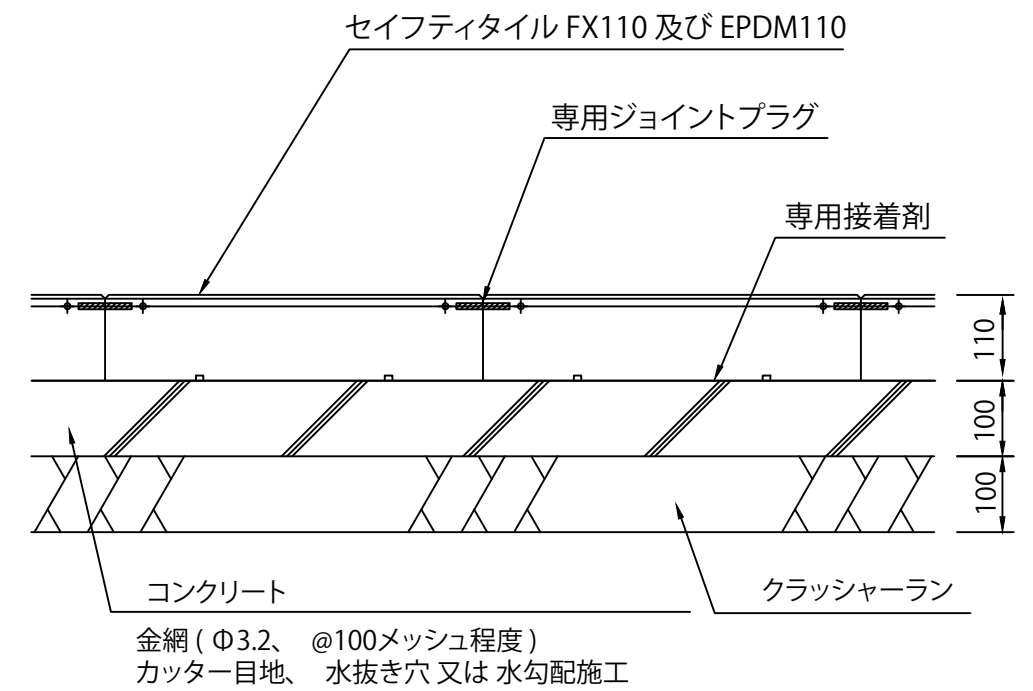
参考施工図 S = 1 / 10
