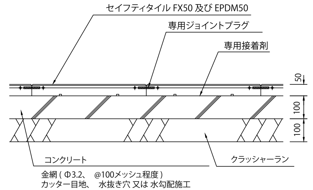
参考施工図 S = 1 / 10
