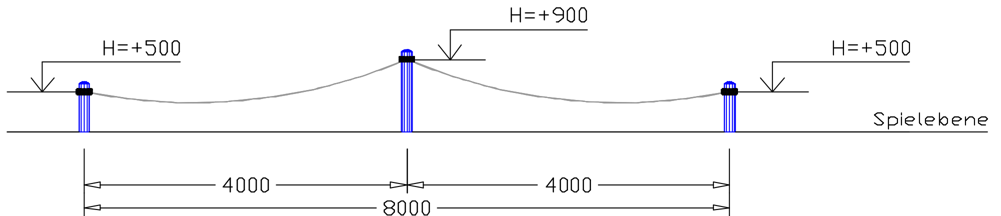
Ansicht, M 1:50
