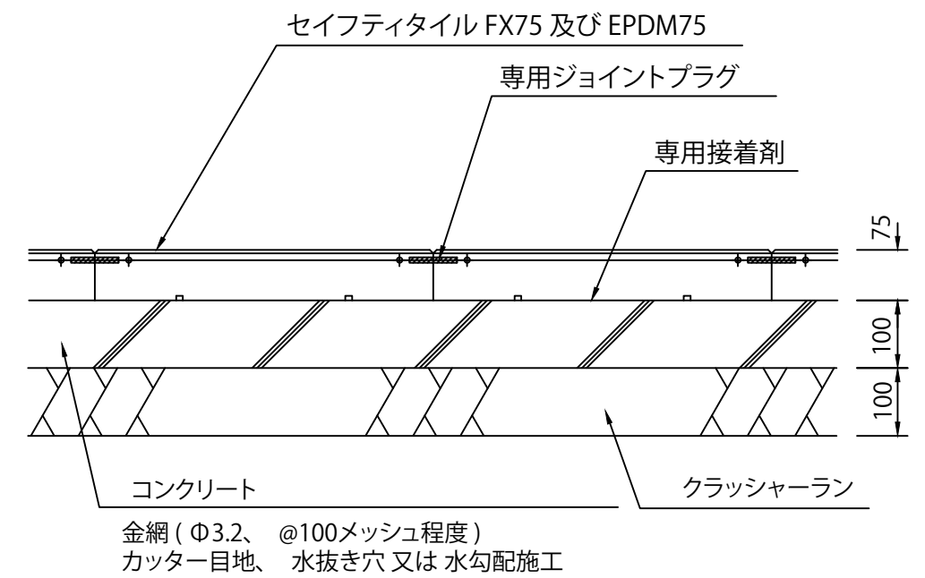
参考施工図 S = 1 / 10
