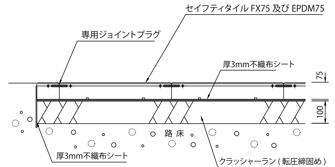
参考施工図 S = 1 / 10
